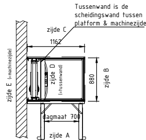
Bovenaanzicht
