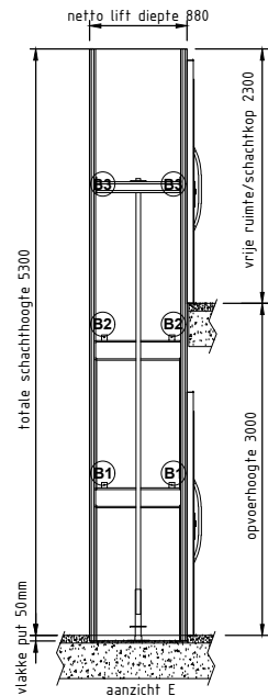
aanzicht E
